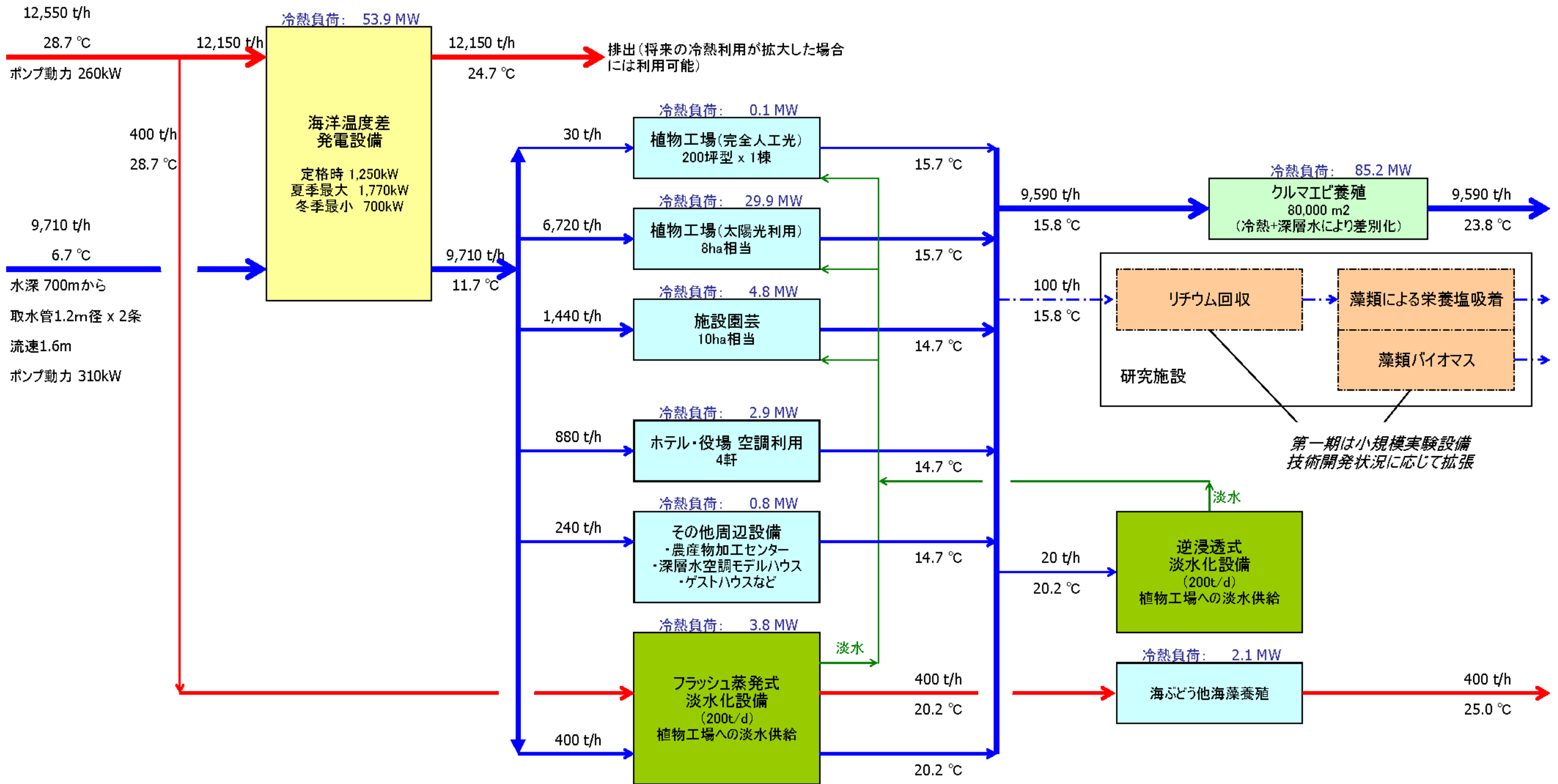
図表 13-1 深層水および表層水のフローと熱物質バランス
